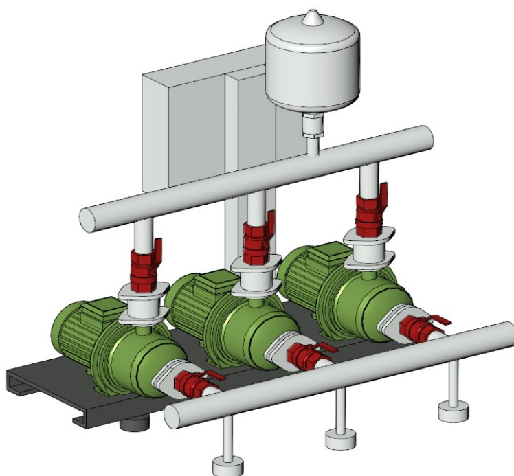
Рис. 4 Трехагрегатная насосная станция на базе горизонтальных центробежных насосов с ручной запорной арматурой
